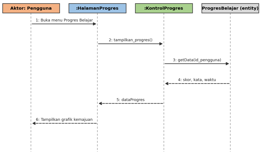
Diagram Sekuens: Melacak Hasil Evaluasi Belajar
