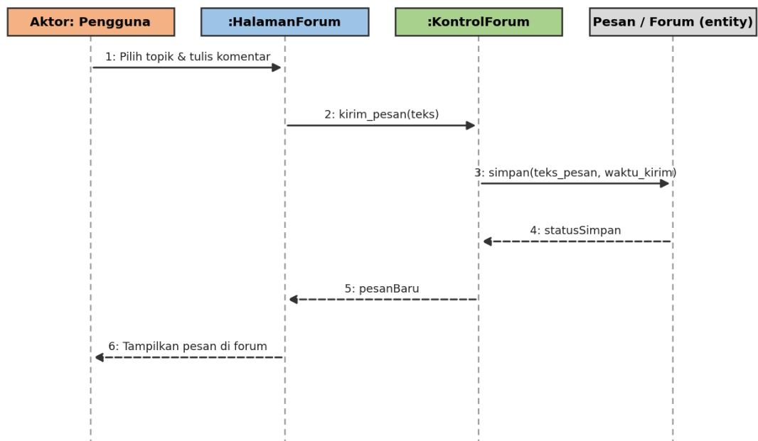
Diagram Sekuens: Mengirim Pesan Teks ke Forum Diskusi
