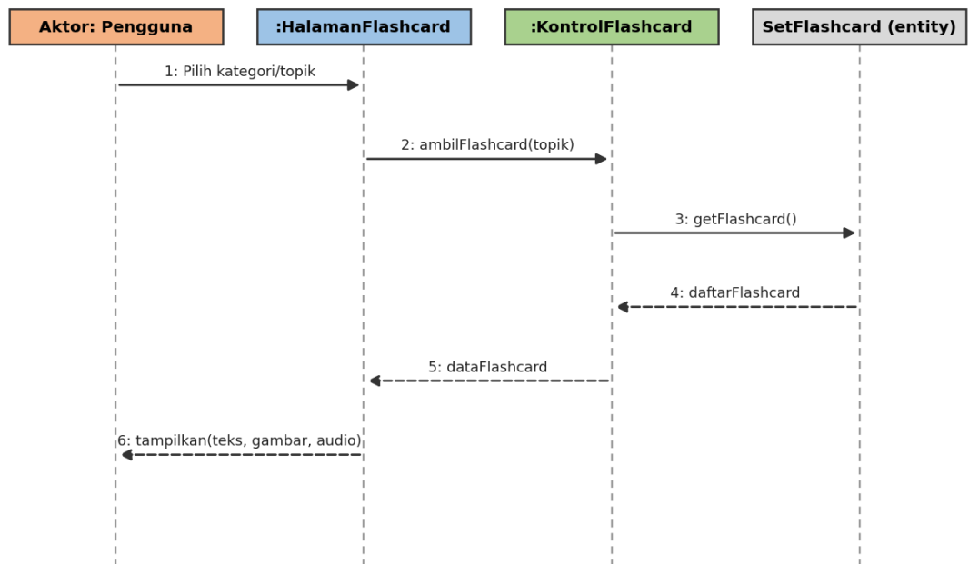
Diagram Sekuens: Menampilkan Flashcard Interaktif
